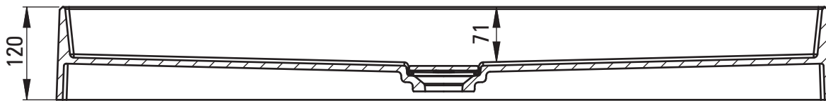
PRZEKRÓJ A-A
